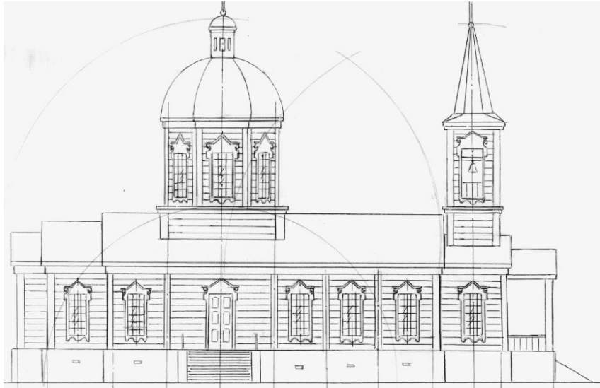
Рисунок 27. Эскиз Свято-Екатерининской церкви (автор И. Л. Коновалов)
