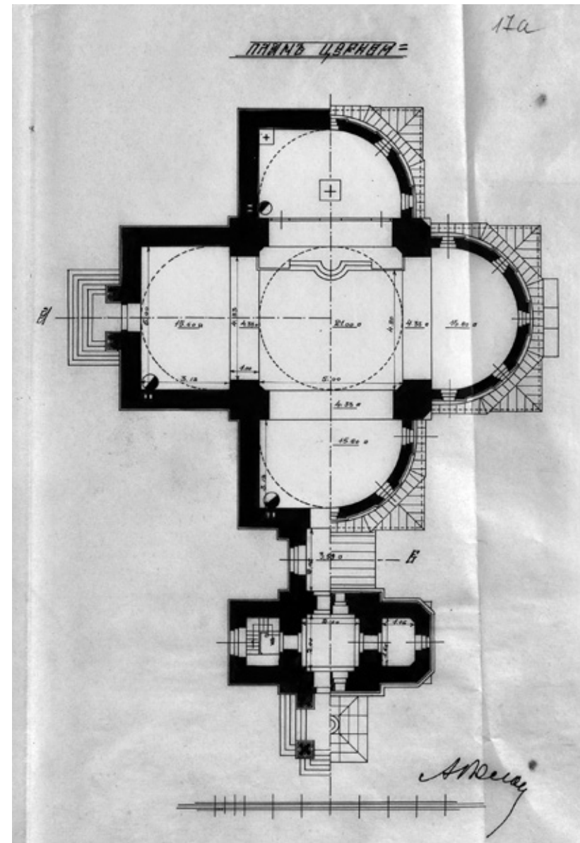
План церкви в с. Корнеевка архитектора А. А. Волошинова. ЦГАСО. Ф. 1. Оп. 12. Т. 2. Д. 4745. Л. 17а
